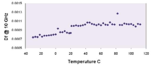
TSM-DS3 : 伴随温度变化的 DF
