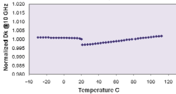
TSM-DS3 : 伴随温度变化的 DK
