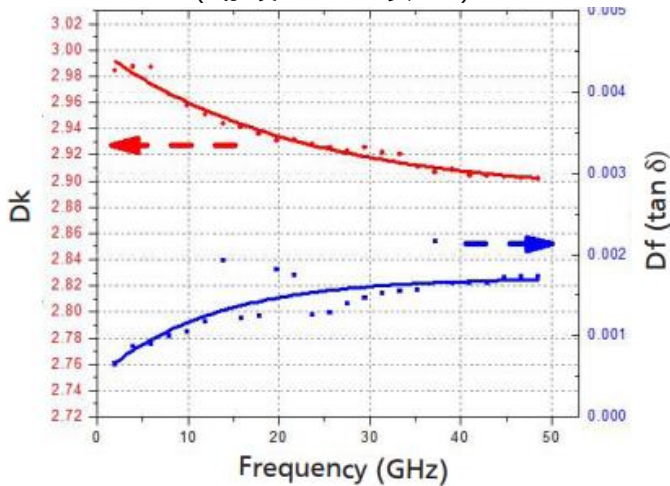
TSM-DS3-0100 上的环形谐振器性能与频率。 (试验设置如第 4 页所示)。
